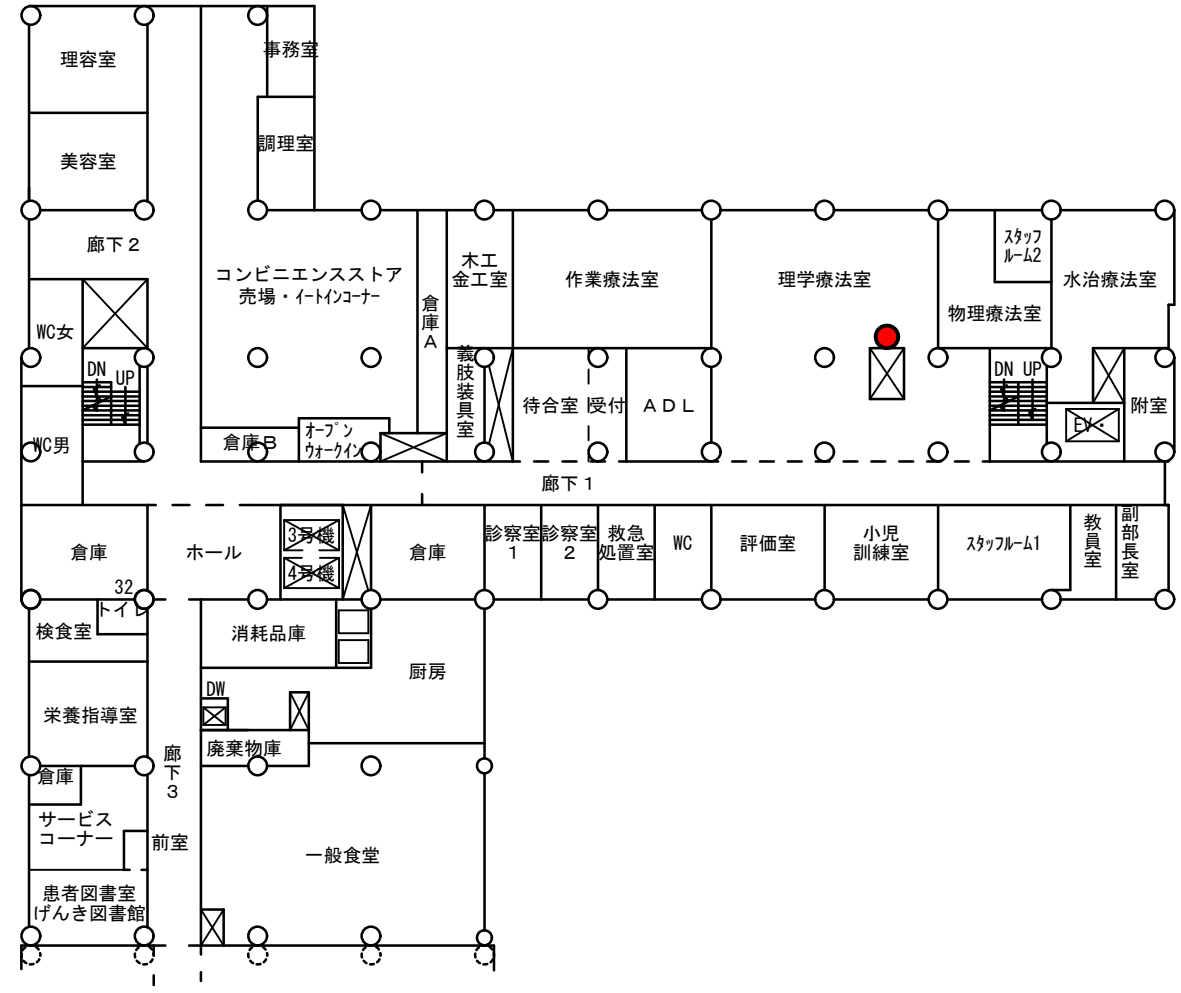
(067) 第二病棟1階平面図 1/400
