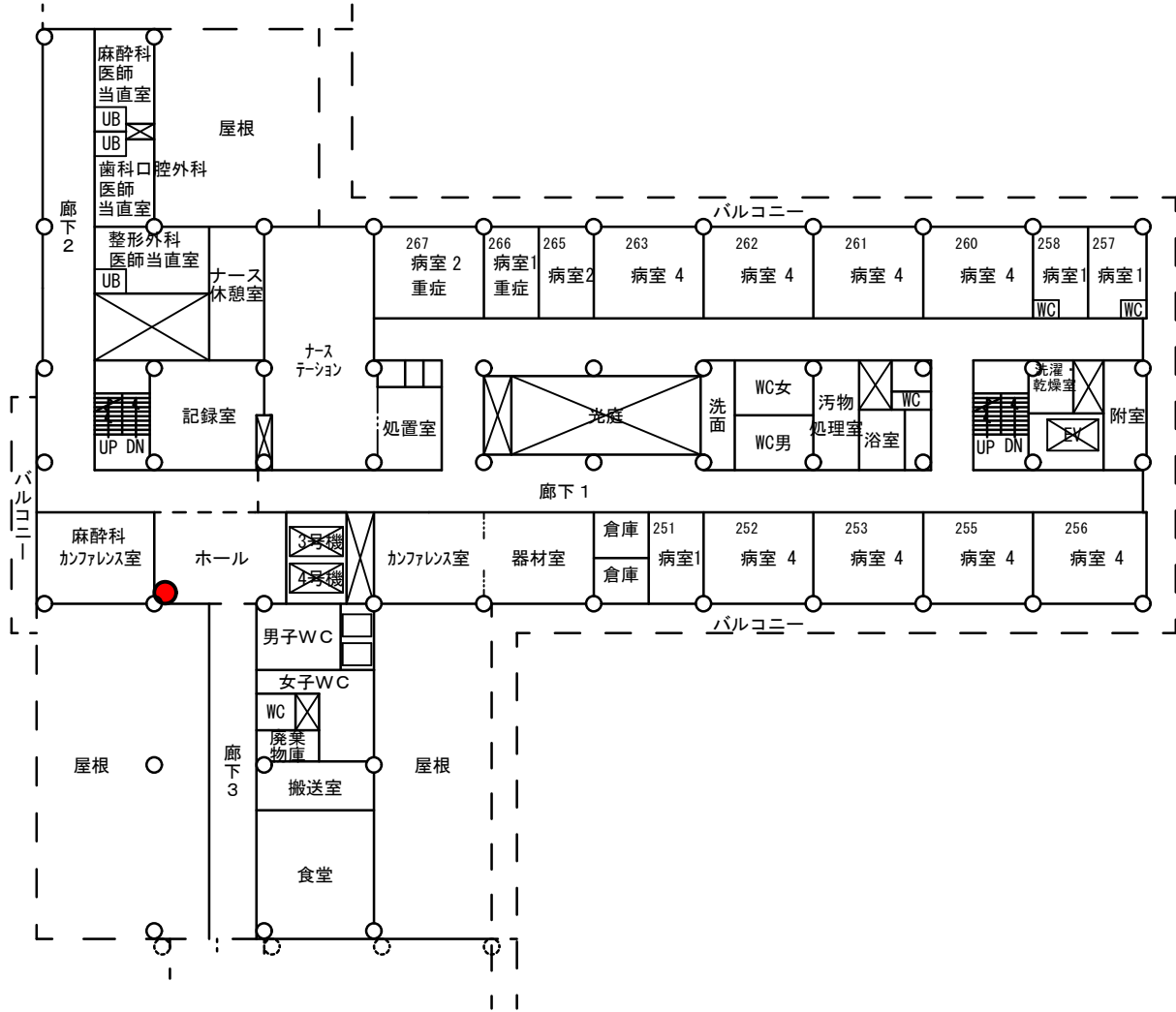
(067) 第二病棟2階平面図 1/400
