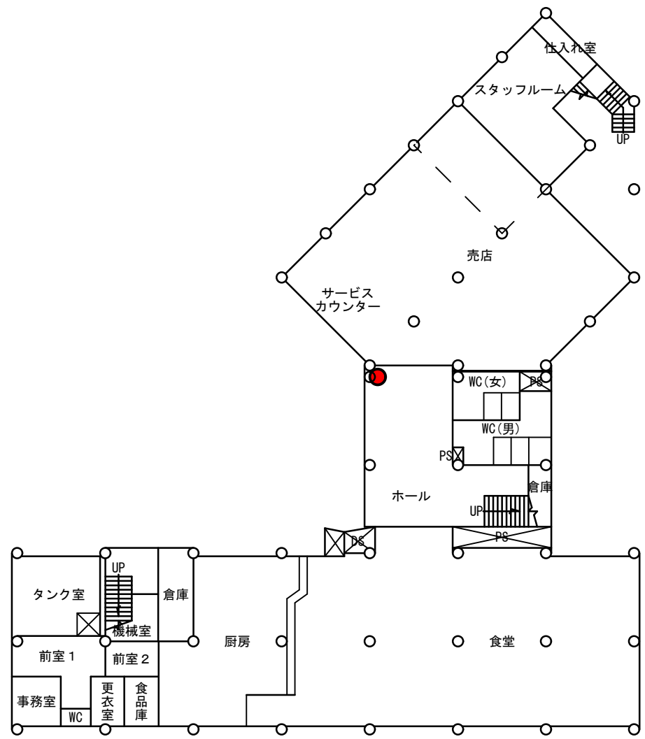
(014) 福利厚生施設 1階平面図 S:1/300
