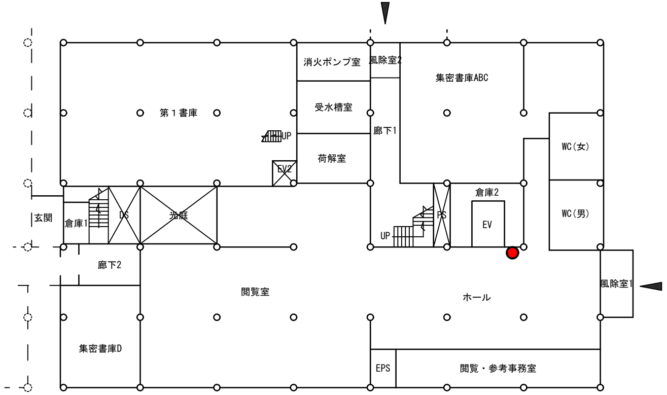
(057) 図書館 1階平面図 S=1/300
