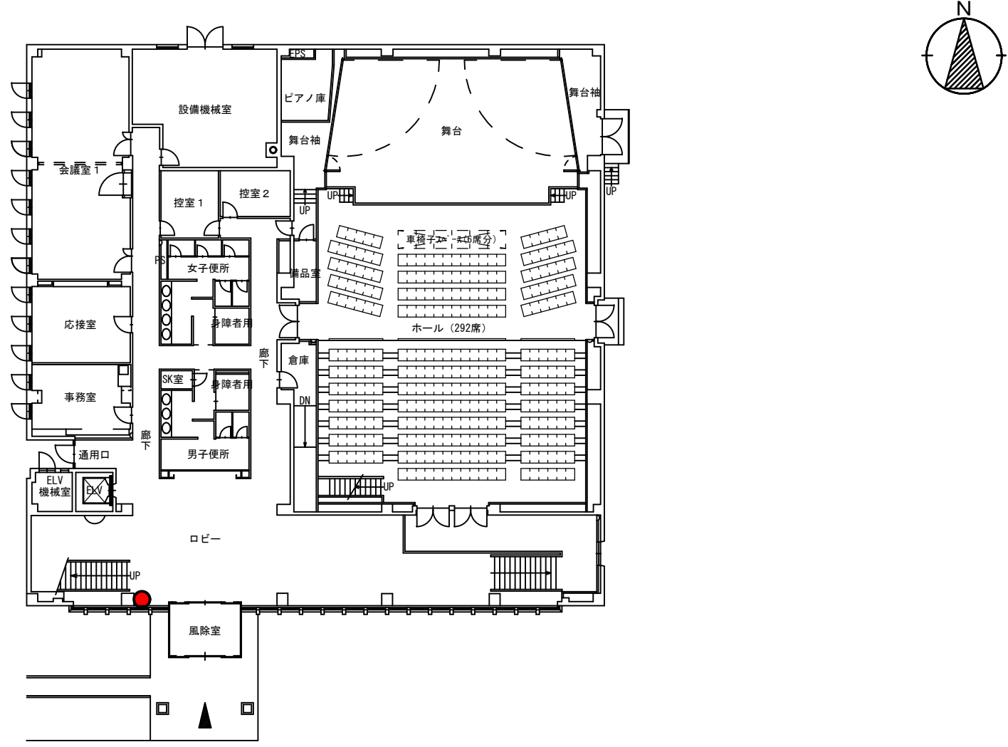
1階平面図 S=1/300
