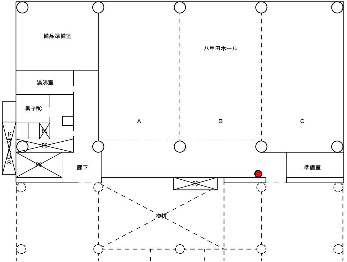
(102) コラボ弘大 8階平面図 S:1/200
