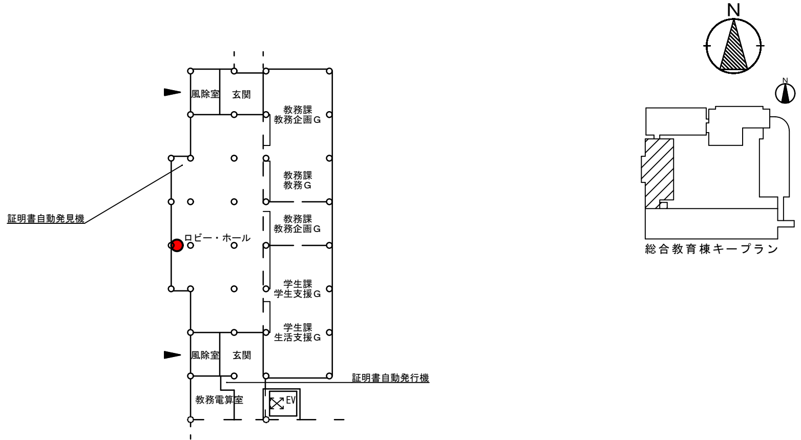
(051) 総合教育棟 1階平面図 S=1/400
