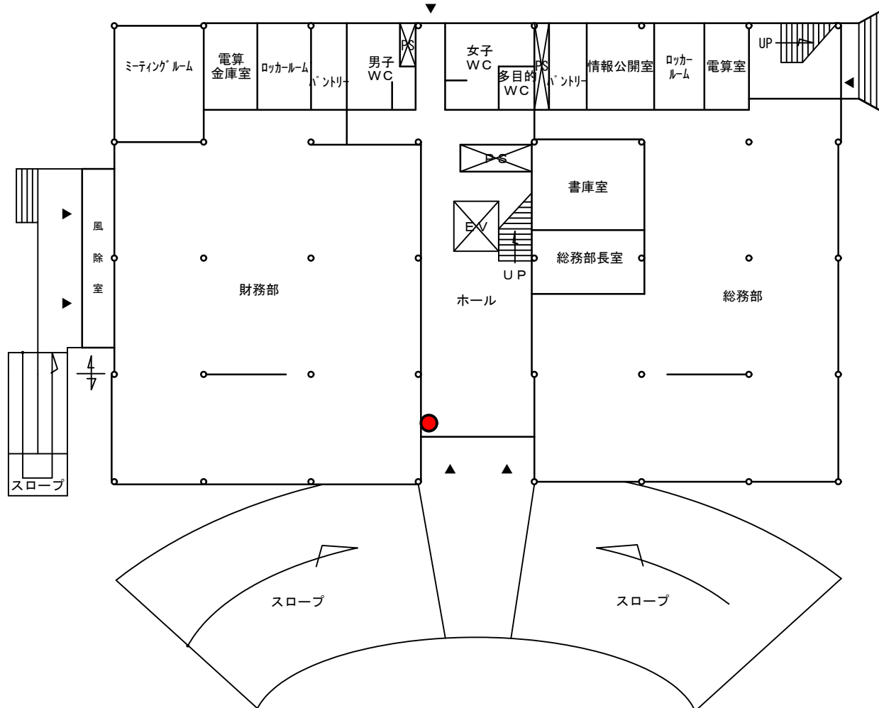
(045) 大学事務局庁舎 1階平面図 S:1/300
